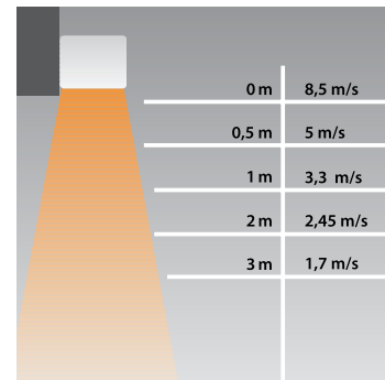
Distancia/velocidad aire
