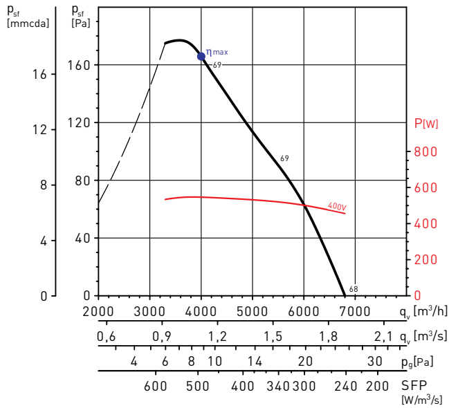
HCBT/4-450/H
